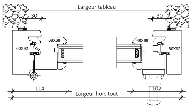
Coupe horizontale
