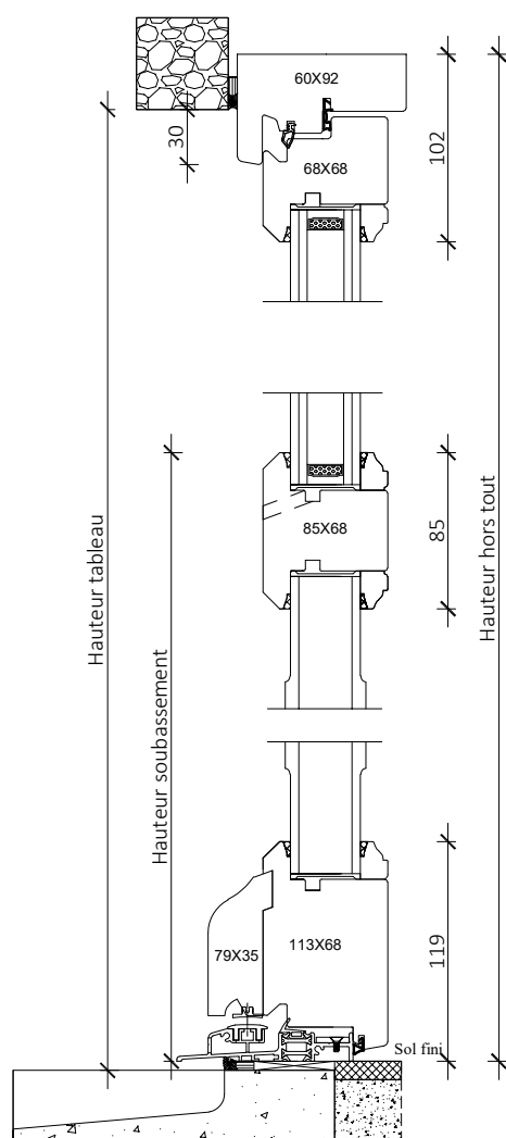
Coupe verticale
