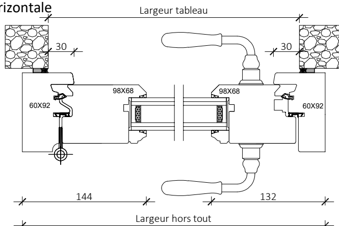
Coupe horizontale
