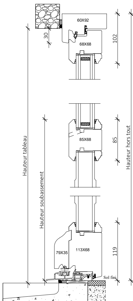
Coupe verticale
