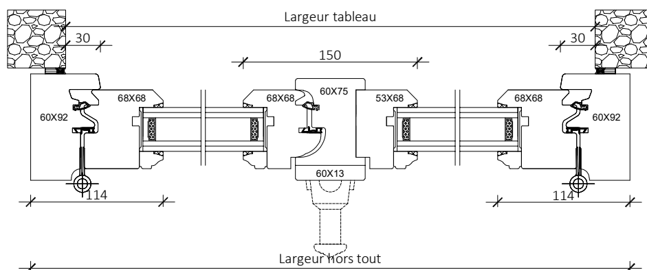
Coupe horizontale
