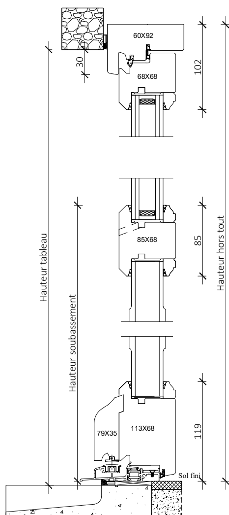
Coupe verticale
