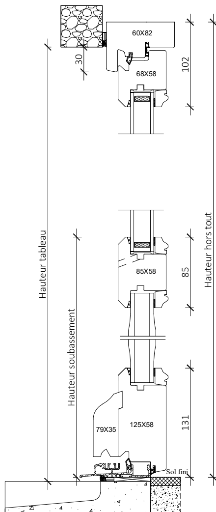
Coupe verticale
