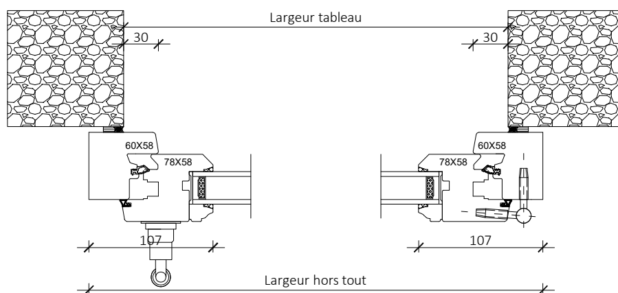
Coupe horizontale
