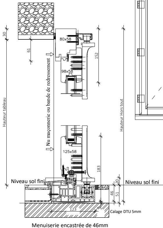
Coupe verticale
